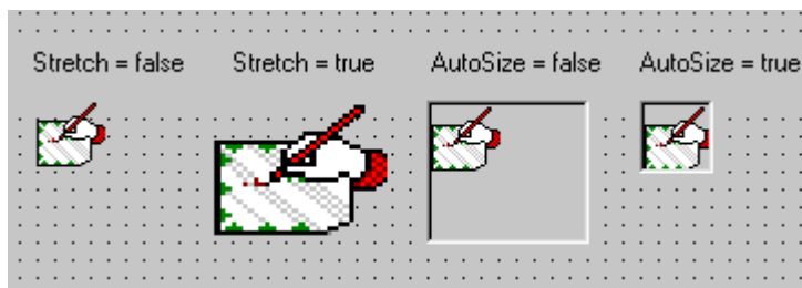
Figura 6.5. Comparación entre image y picture con bitmaps .
