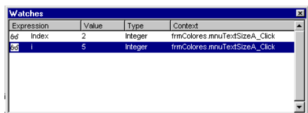
Figura 2.18. Ventana Watches .
