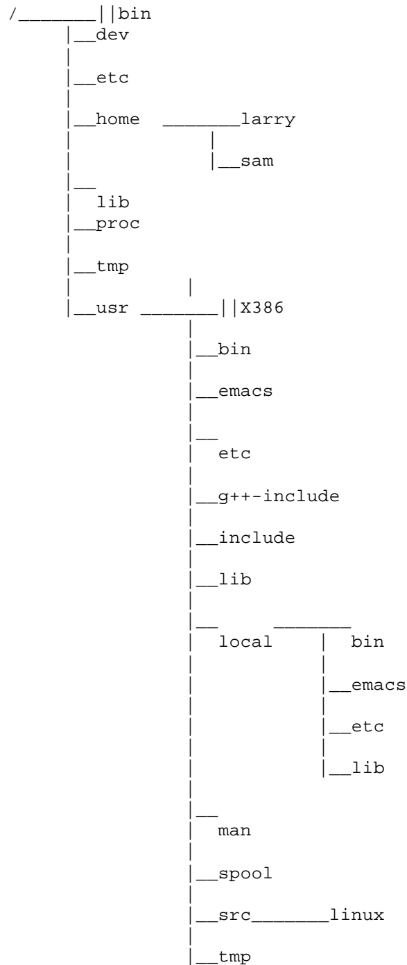
Figura 3.1: Típico árbol de directorios Unix (resumido).
